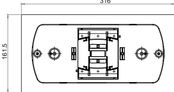
SafeLite 20m mennyezeti süllyesztőkeret
