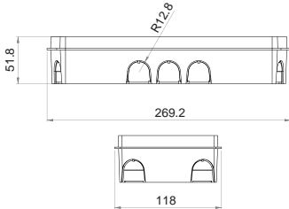
SafeLite 20m fali süllyesztő doboz
